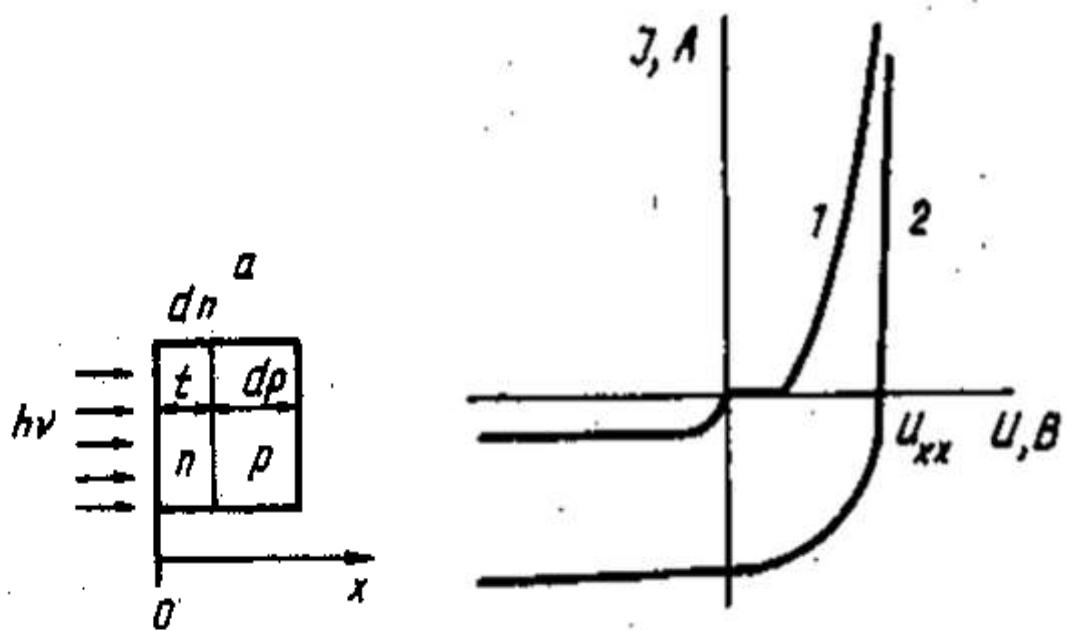
4-rasm.Yupqa p-n- o'tishli fotoelement va fotodiodning volt-amper xarakteristikasi
